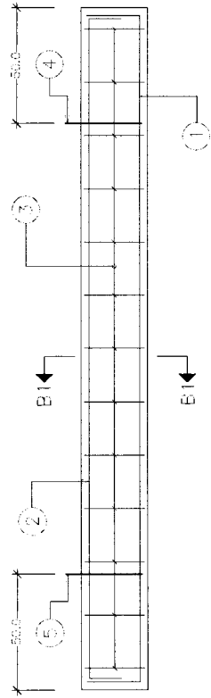
آرماچور بندی تیر میانی
